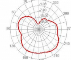
2500.000MHz H
