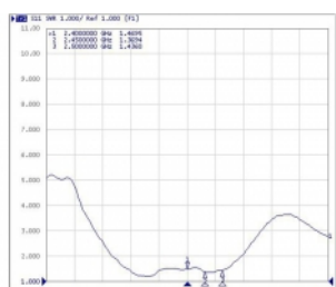
2400.000MHz E2
